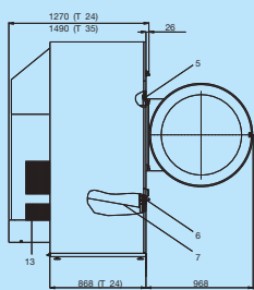
ZEZADU T 24 35 (PLYNOVÝ MODEL)
