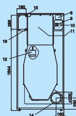
ZEZADU T 24 35 (PARNÍ MODEL)
