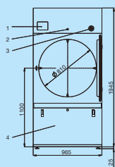
ZEZADU T 24 35 (PARNÍ MODEL)
