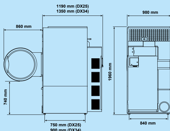
Boční pohled DX 25 34
