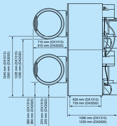
Boční pohled DX 13/13 20/20
