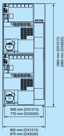
Zadní pohled DX 13/13 20/20
