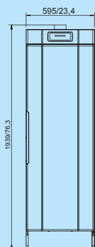
Čelní pohled
